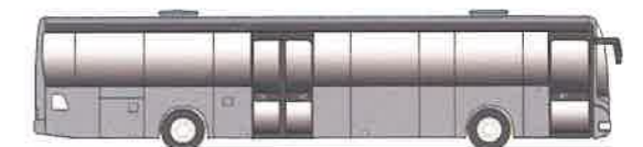
12,8m 1 porta anteriore 800 mm e 1 porta centrale 1200 mm
