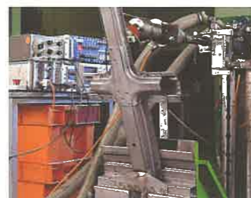
Tests endurance montant de baie.
