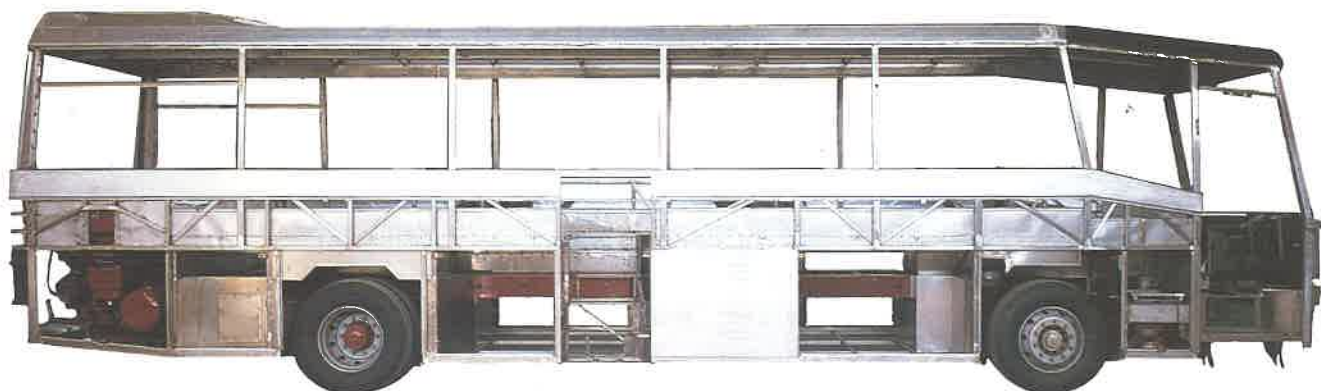
Struttura in acciaio inox
