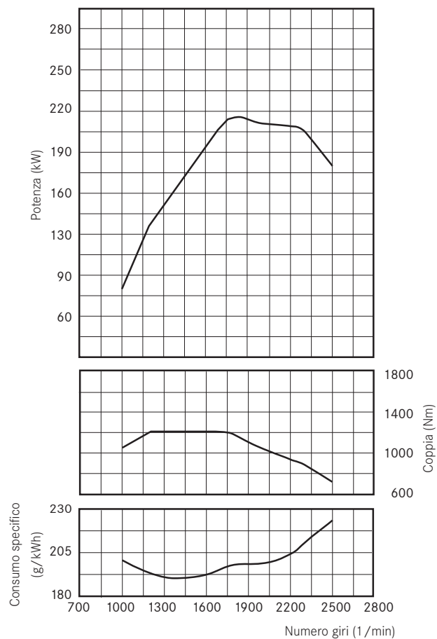
Motore OM 936 h/OM 936 (Euro VI D)
