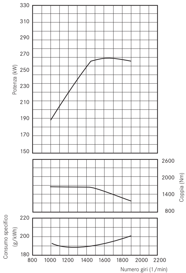
Motore OM 470 (Euro VI D)
