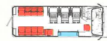
Posti 10+3+1
